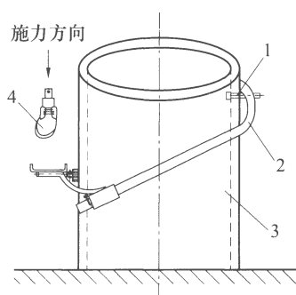
1—限位装置；2—登杆脚扣；3—模拟电杆；4—鞋模
