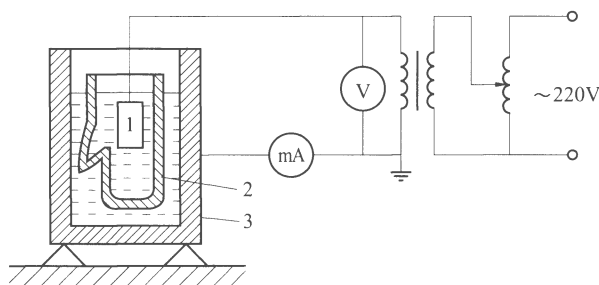
图 B.4 辅助型绝缘手套试验接线图
